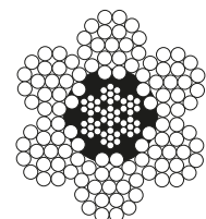
6 x 19
